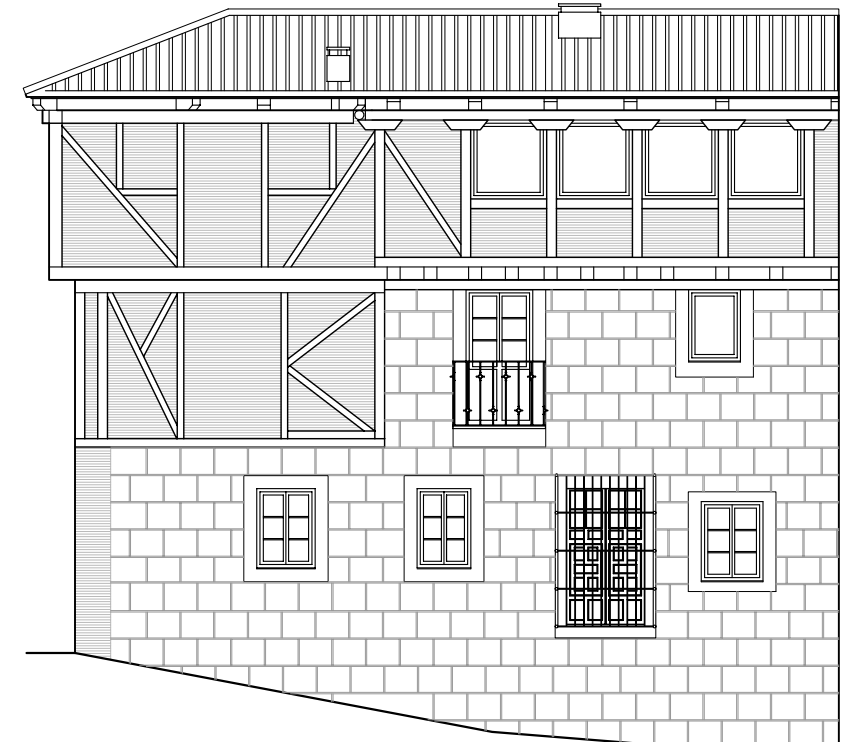
ALZADO C/ JUDERIA NUEVA
