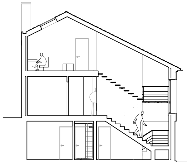
SECCIÓN TRANSVERSAL
