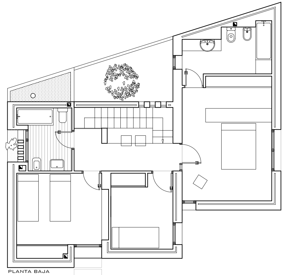
PLANTA BAJA
