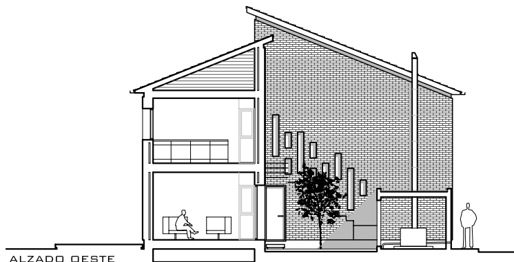
ALZADO OESTE
