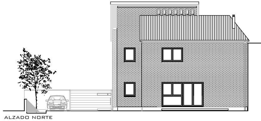
ALZADO NORTE
