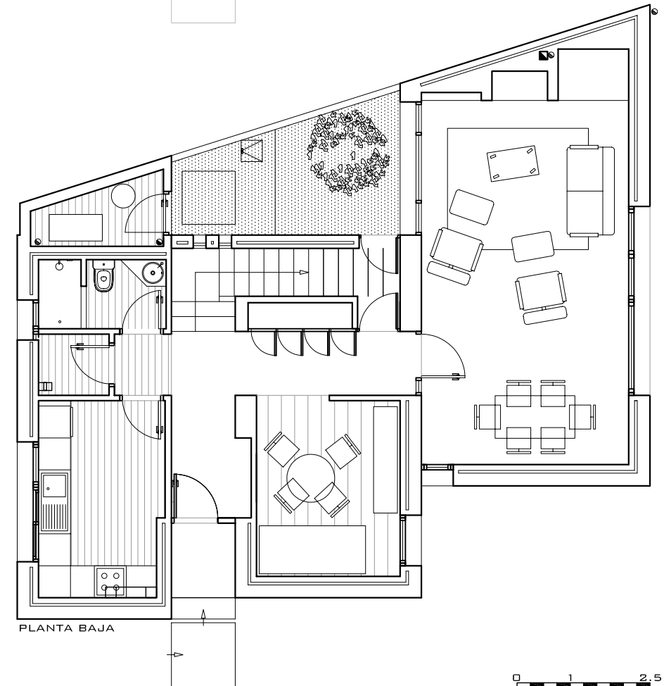
PLANTA BAJA
